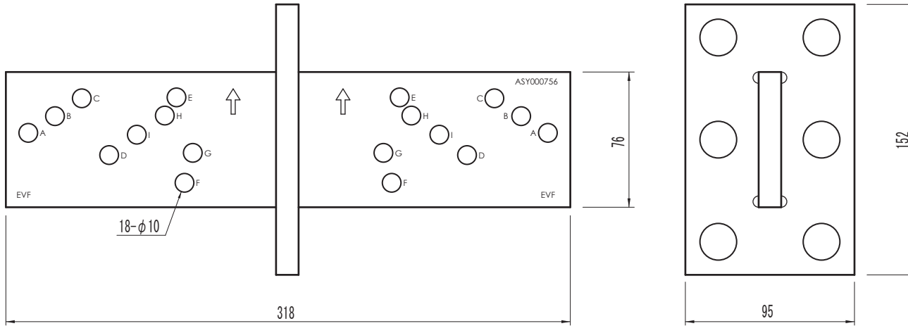
■EVF ロングリギングプレート (3.33 kg) x2
