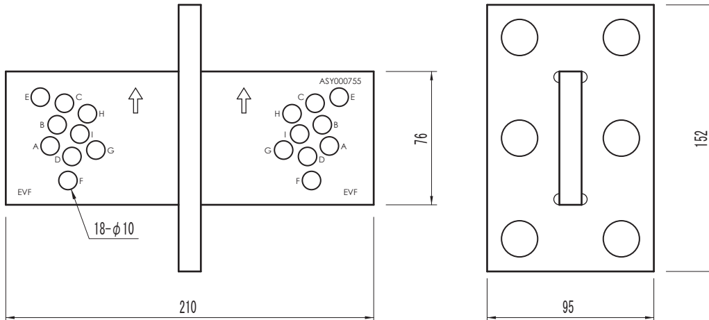
■EVF ショートリギングプレート (2.53 kg) x2
